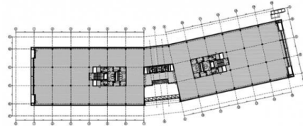
Typické patro / Typical floor
